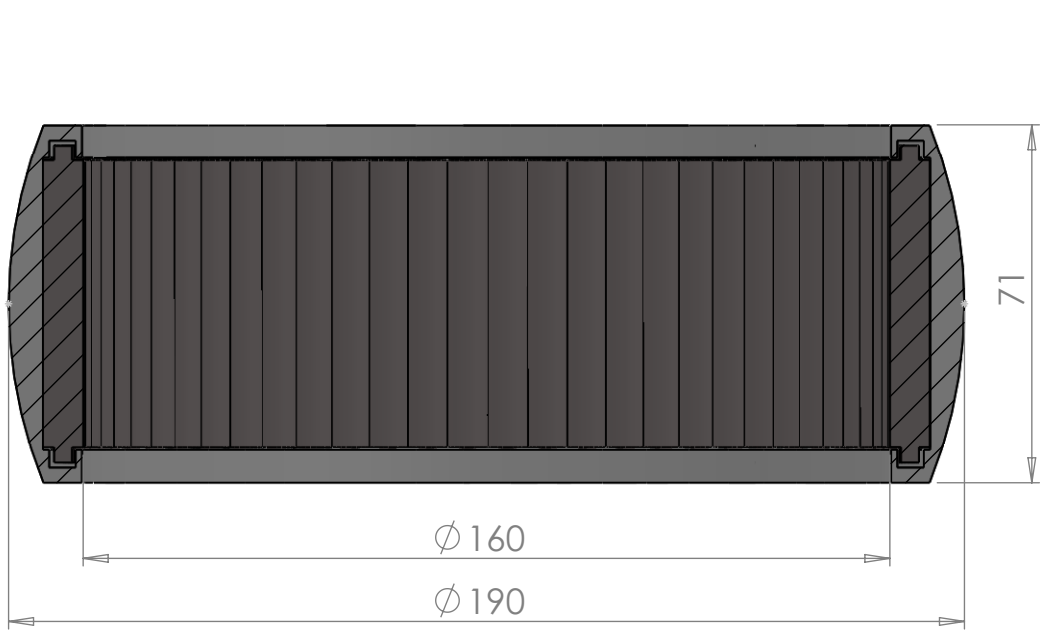
SECTION A-A SCALE 1 : 1.5
