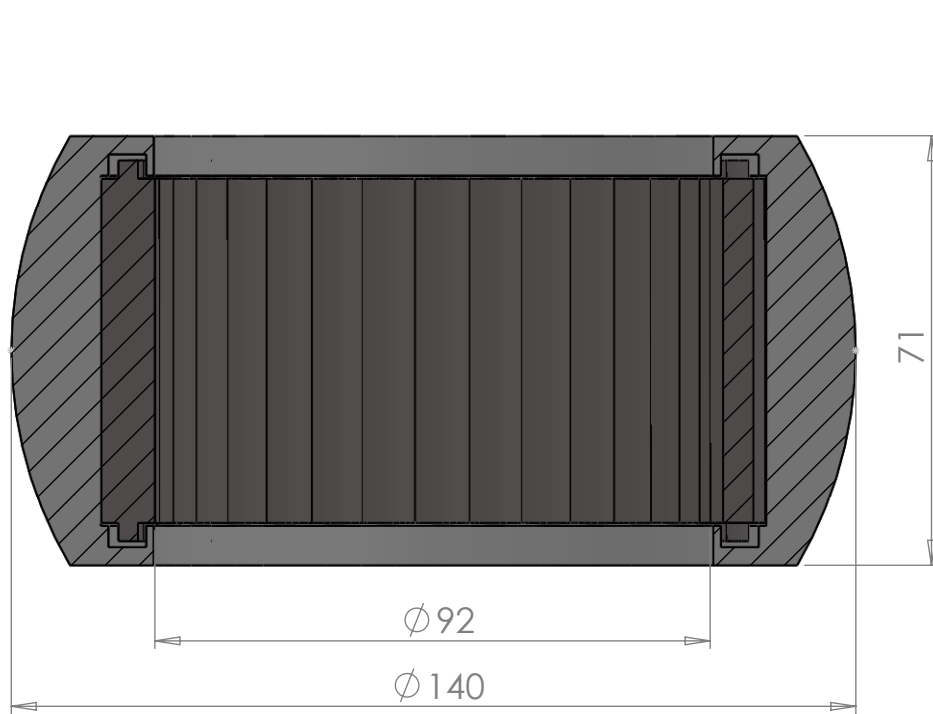
SECTION A-A SCALE 1 : 1.25
